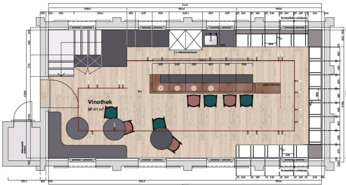
Projekt der Firma Gehri AG, Aarberg – Grundriss Obergeschoss Vinothek
